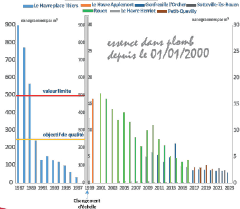
Evolution des concentrations de plomb
